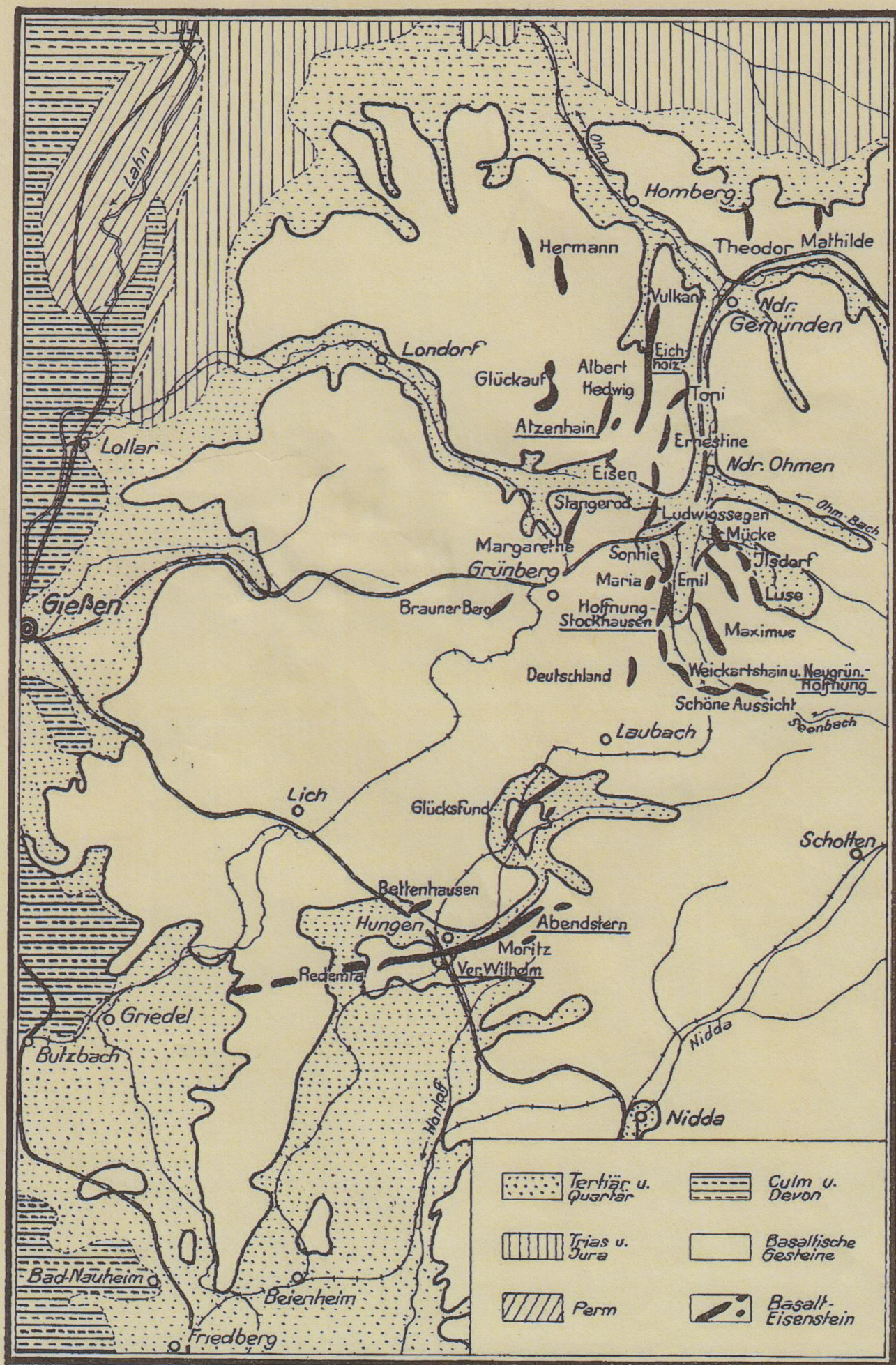
Fig. 19. Die Basalteisenerzlagerstätten im Vogelsberg (nach Witte)
